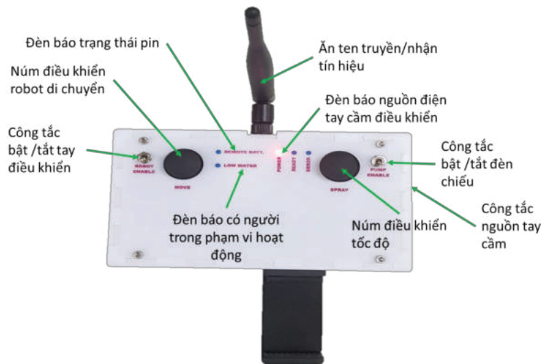
Hình 2: Mô tả tính năng tay cầm điều khiển
